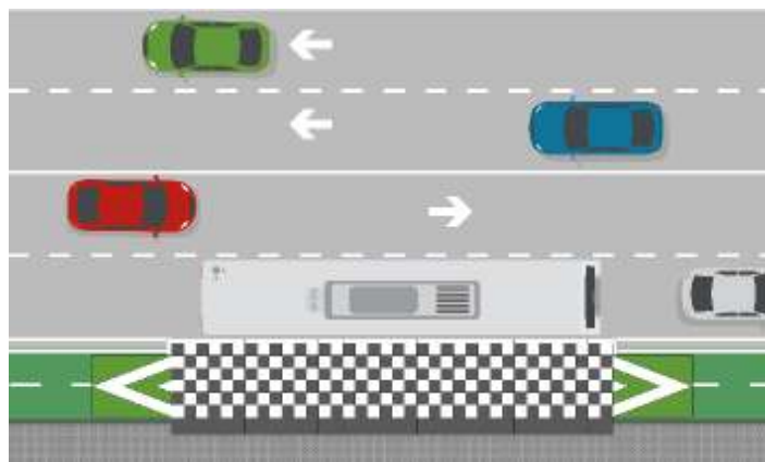
PLATEFORME AVEC PISTE CYCLABLE INTÉGRÉE BUS DE 12m (17,5 m x 3 m).
