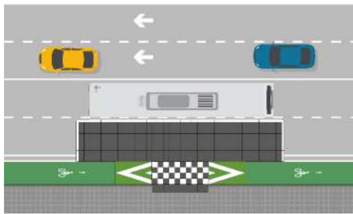
PLATEFORME AVEC PASSERELLE D'ACCÈS ET PISTE CYCLABLE INTÉGRÉE BUS DE 12m (12,87 m x 4,4 m).
